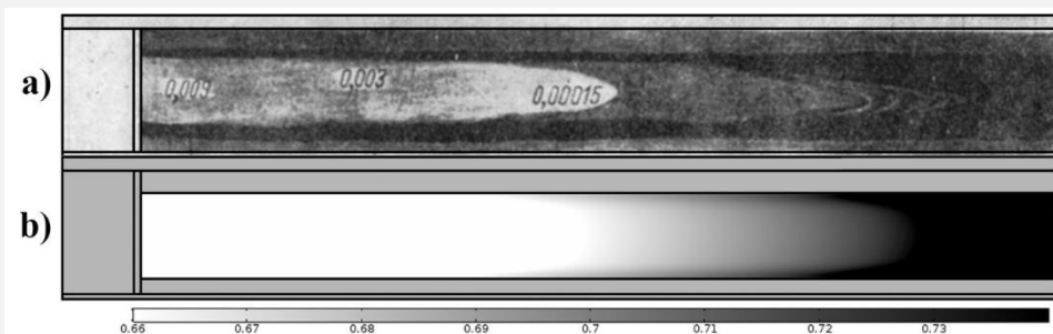
Рисунок 4. Сравнение изменения степени окисления: (а) экспериментальные данные, отражающие распределение концентрации восстановителя вдоль контейнера [16]; (б) модельное распределение восстановителя, полученное в результате численного моделирования.
