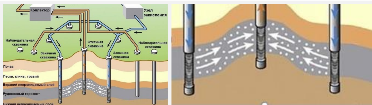
Рисунок 1. Схема извлечения урана методом подземного скважинного выщелачивания.
