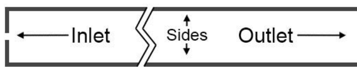
Рисунок 3. Схема лабораторного контейнера для имитации образования урановых ролл-фронтов [16].
